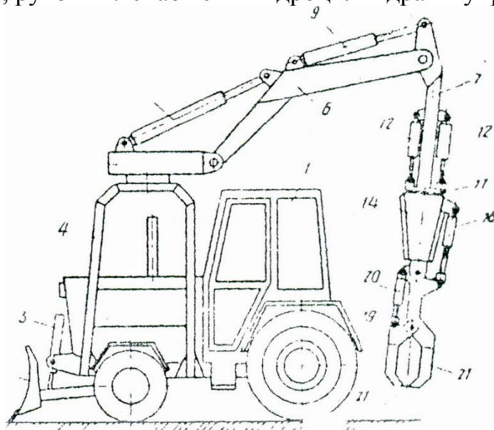
Рисунок 1. Общий вид строительного манипулятора
