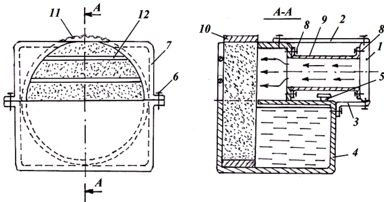
Рисунок 1. устройство для увлажнения воздуха производственной среды: 1 – дефлектор; 2,3 – крепления; 4,7 – нижняя и верхняя стенки корпуса; 5 – крышка горловины; 6;8 – винты; 9 – патрубок; 10 – пористый цилиндр; 11 – рифление
