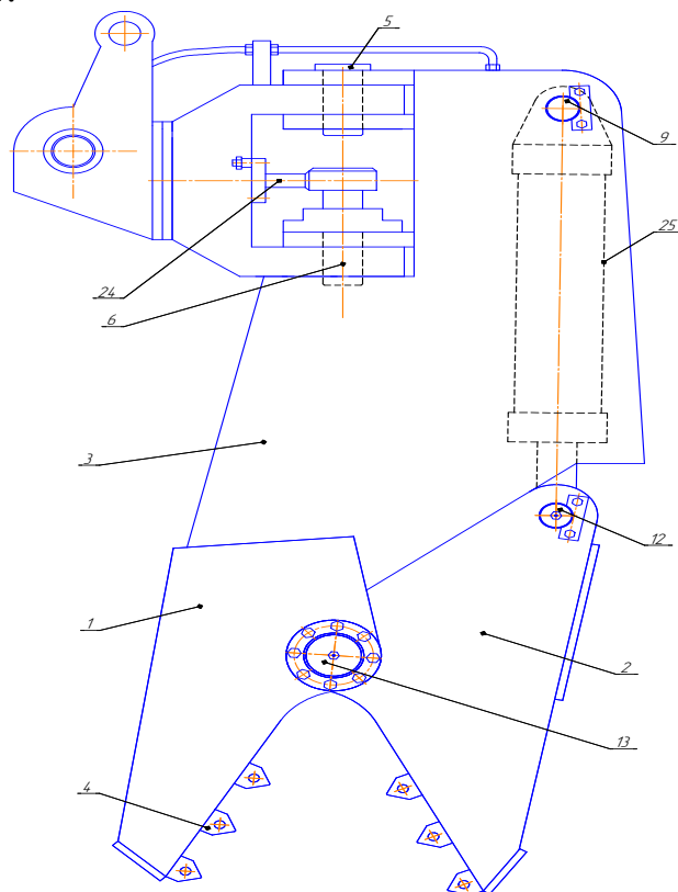
Рисунок 6. Рабочее оборудование для захвата и разрушения строительных конструкций
