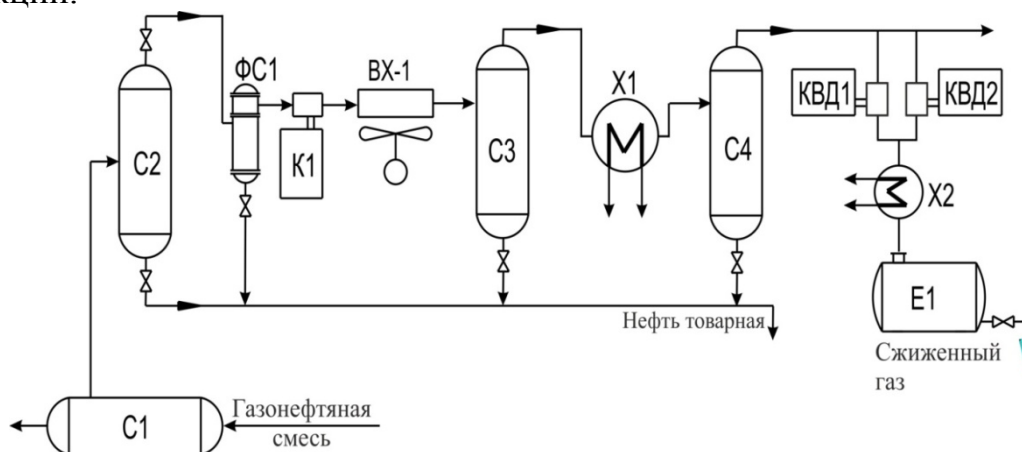
Рисунок 1. Технологическая схема установки получения легких жидких углеводородов (пропан, бутан, пентан).
