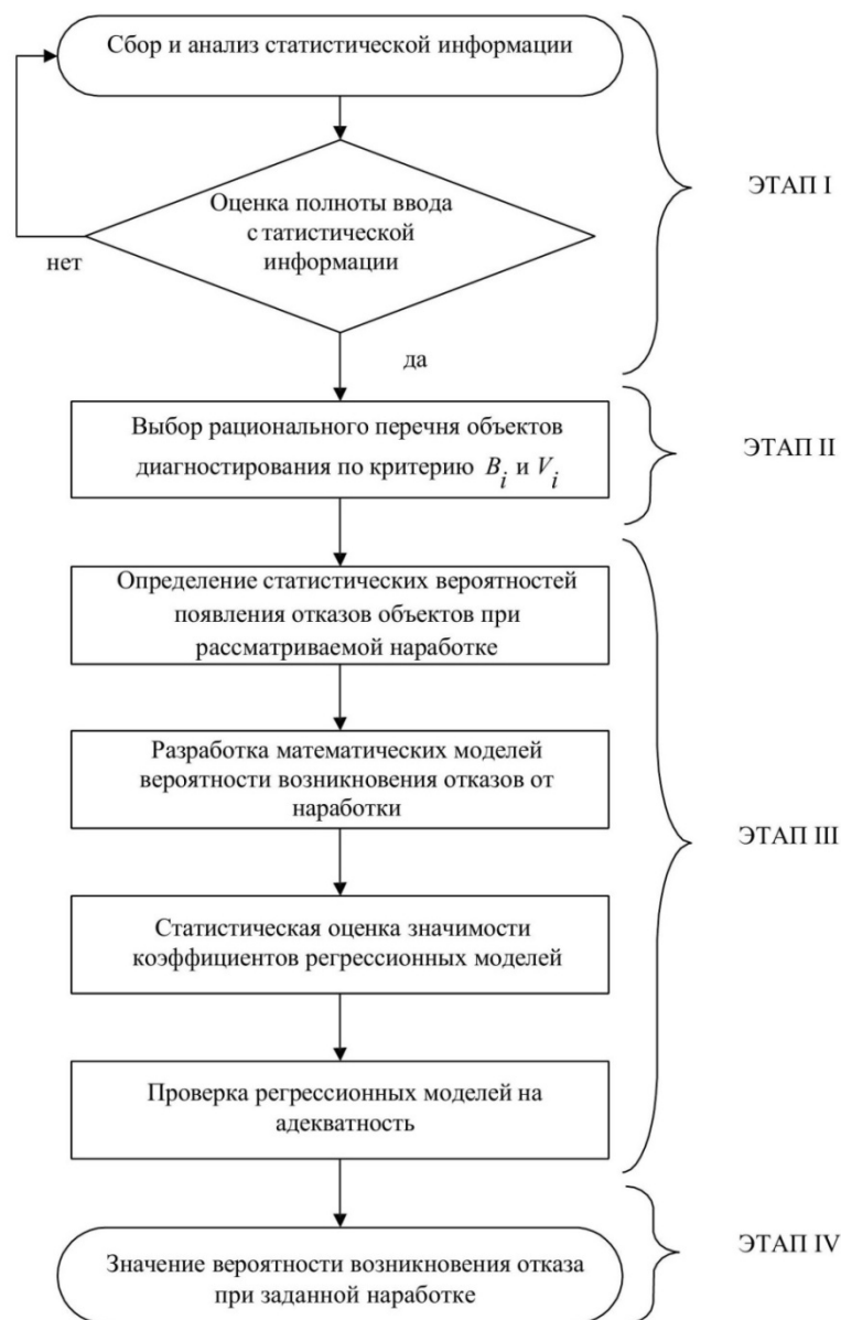
Рисунок 1. Алгоритм прогнозирования технического состояния подвижного состава
