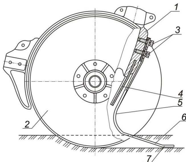
Рисунок 2. Усовершенствованный сошник
