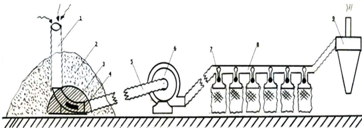
Рисунок 1. Кормоизмельчитель «Шмель»: 1 - «Дыхательная» труба; 2 - сырьё; 3 - камнеуловитель; 4- инжектор; 5 - гибкий пневморукав; 6 - дробилка; 7 - клапан; 8 - мешконабиватель; 9- циклон пылеуловитель
