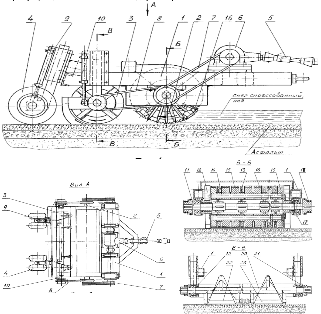
Рисунок 1. Устройство очистки от наледи и спрессованного снега
